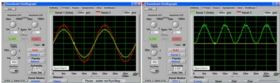
Ohmsche Last: Strom-, Spannungsverlauf (links) und Leistungsverlauf (rechts)
