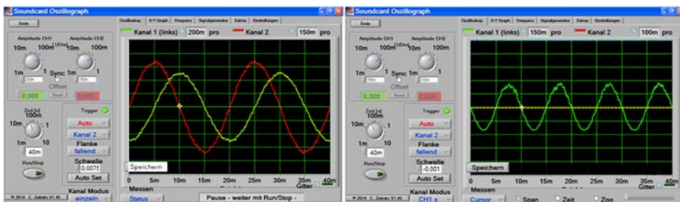
Induktive Last: Strom-, Spannungsverlauf (links) und Leistungsverlauf (rechts)
