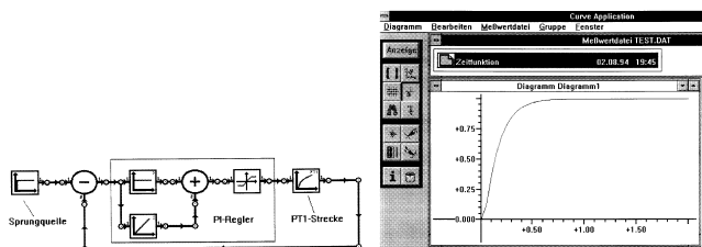
Grafische Eingabe einer Regelkreises in einer Windows-Oberfläche und Auswertung einer Sprungantwort mit BloSIM
