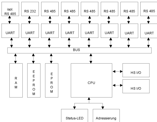
Bild 1: Blockschaltbild der Kreuzschienensteuerung (KSS)
