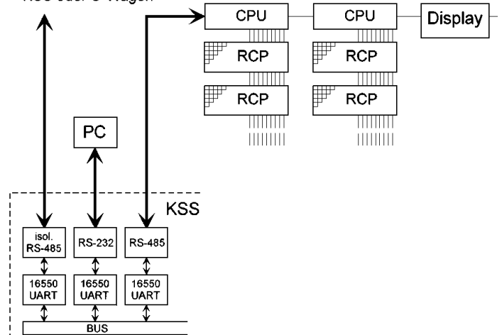
Bild 2: Komponenten
